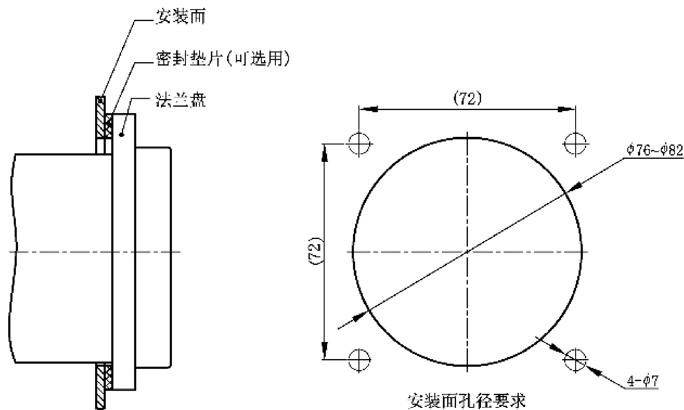
图 6 前安装示例
