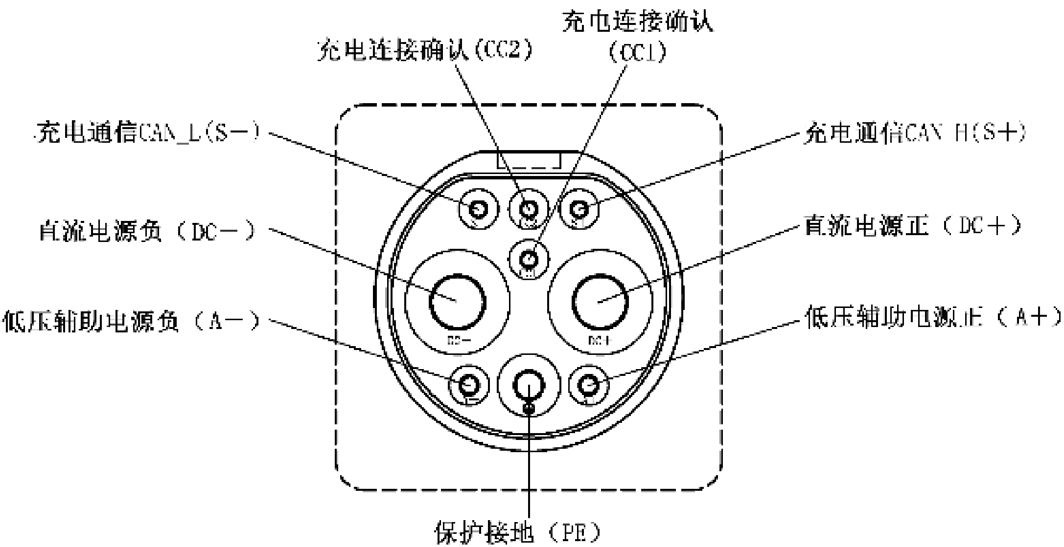
图 2 车辆插座连接界面与触头布置
