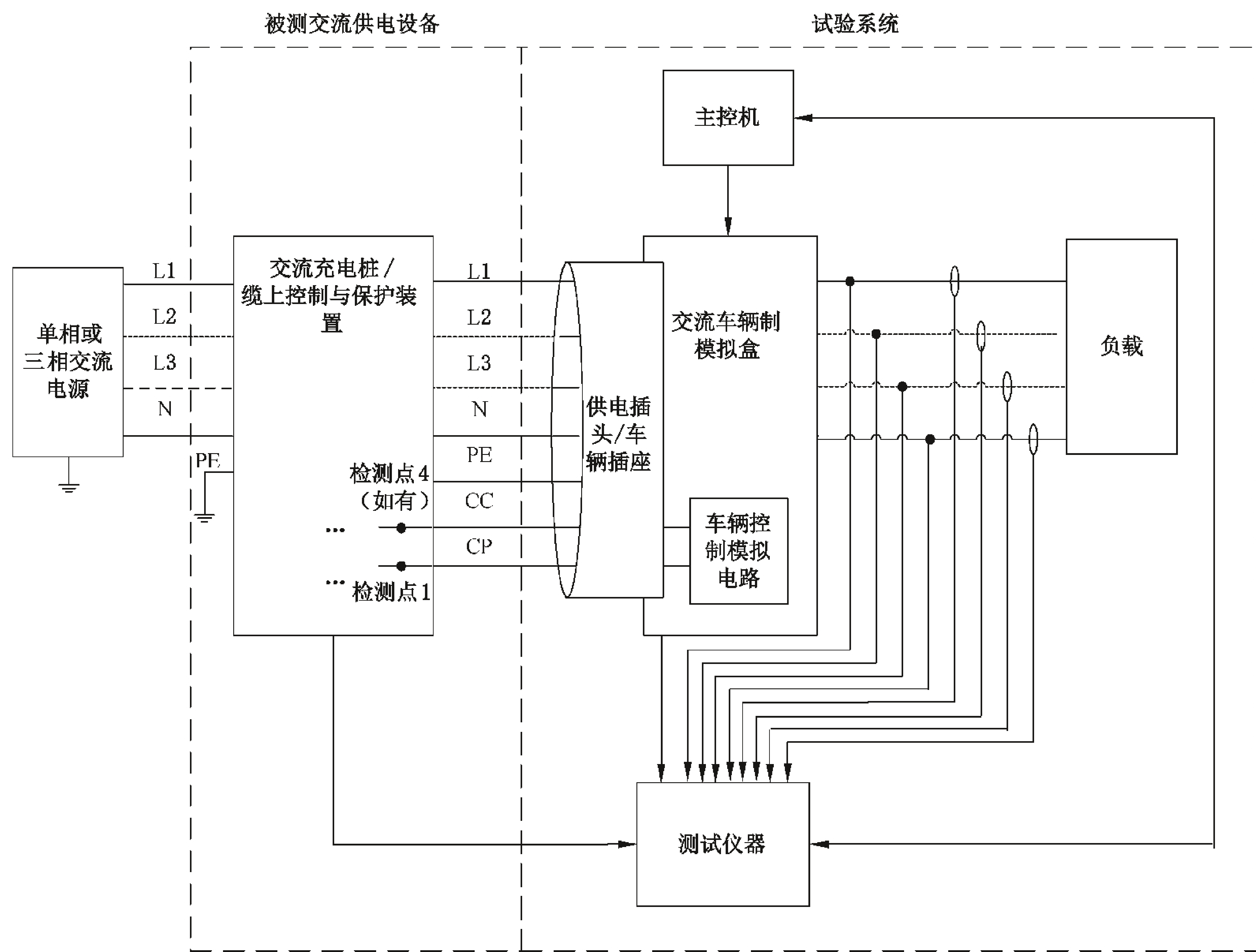
图3 交流供电设备试验系统
