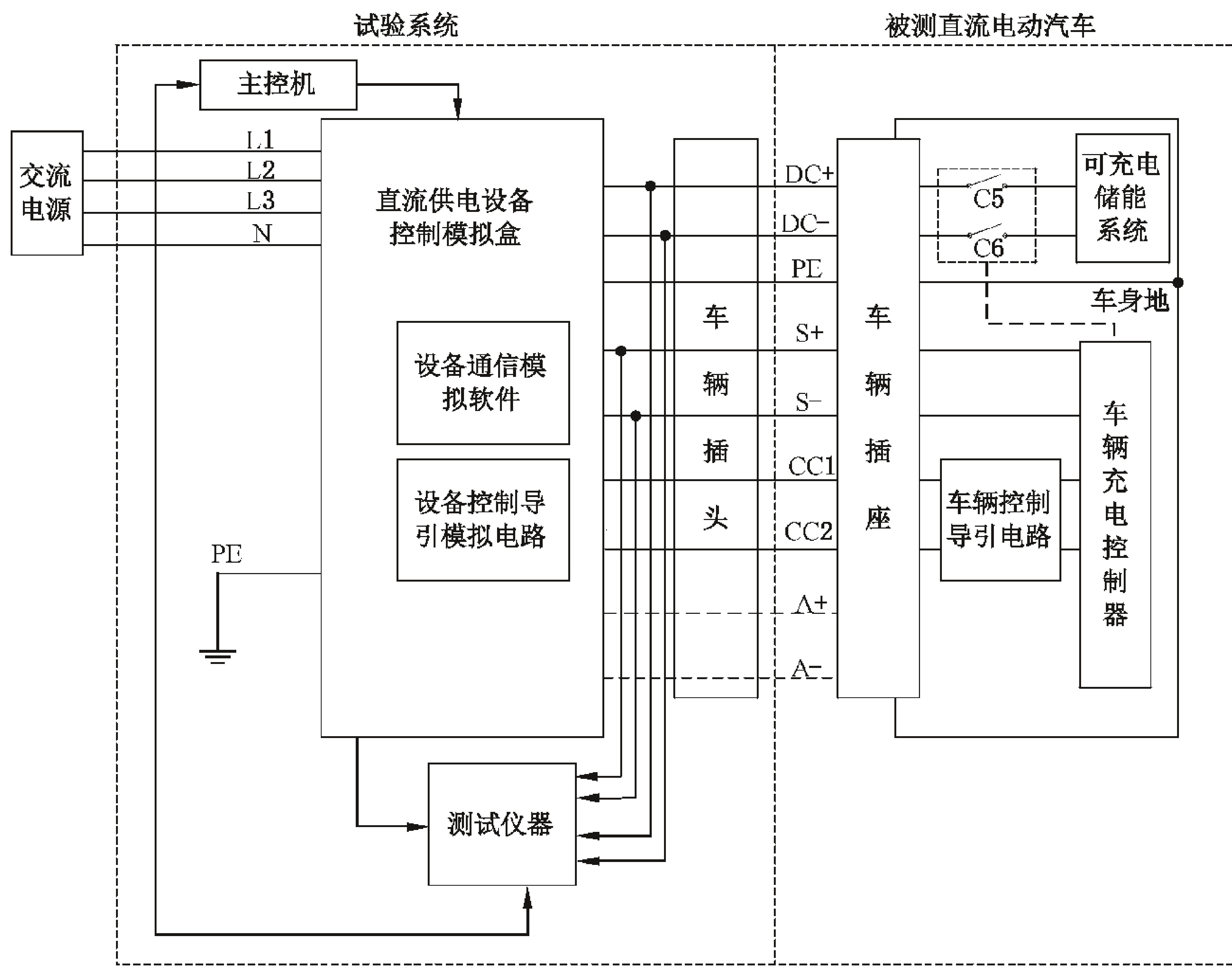
图 6 电动汽车直流充电试验系统结构
