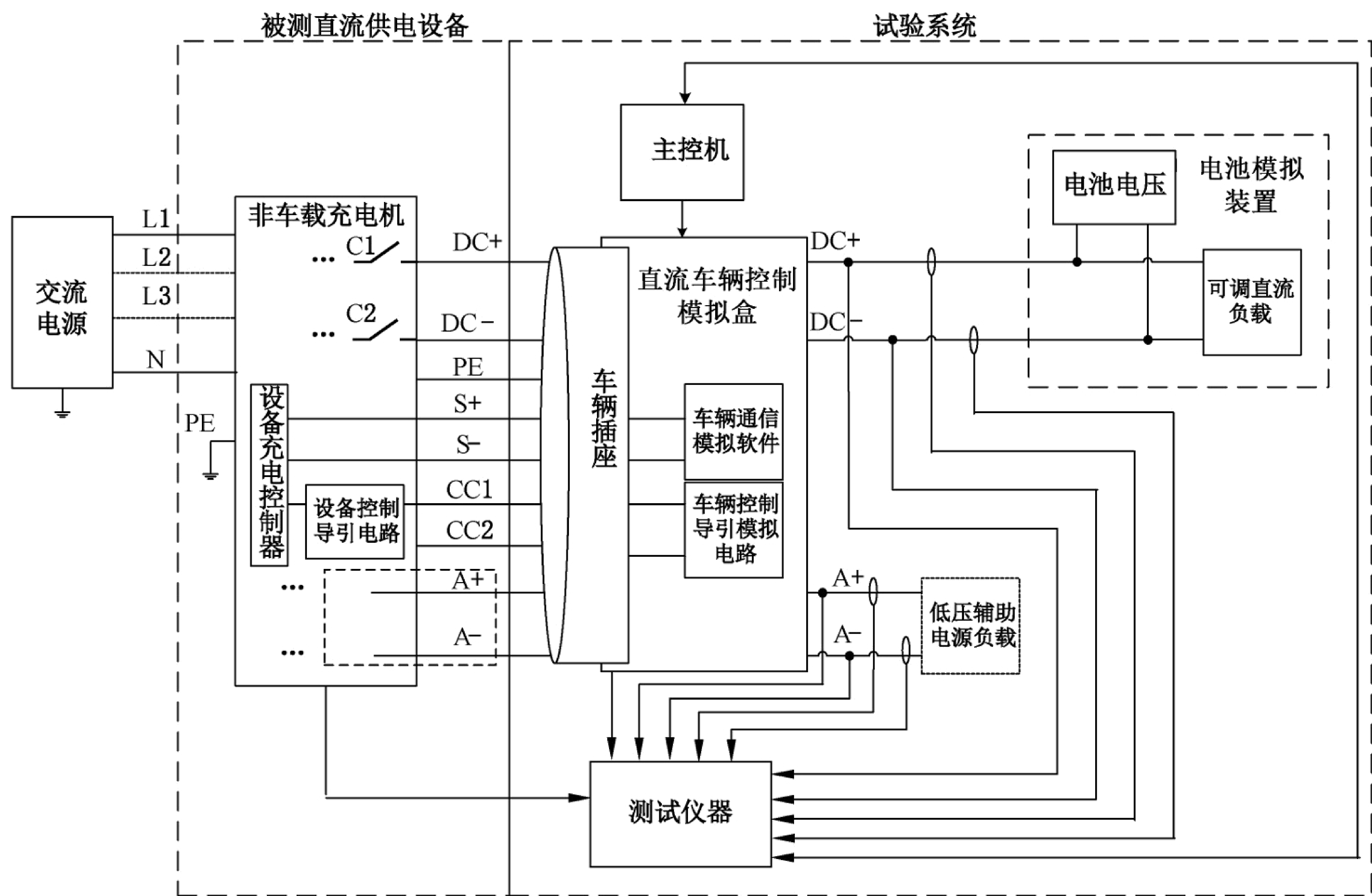
图 5 直流供电设备试验系统结构
